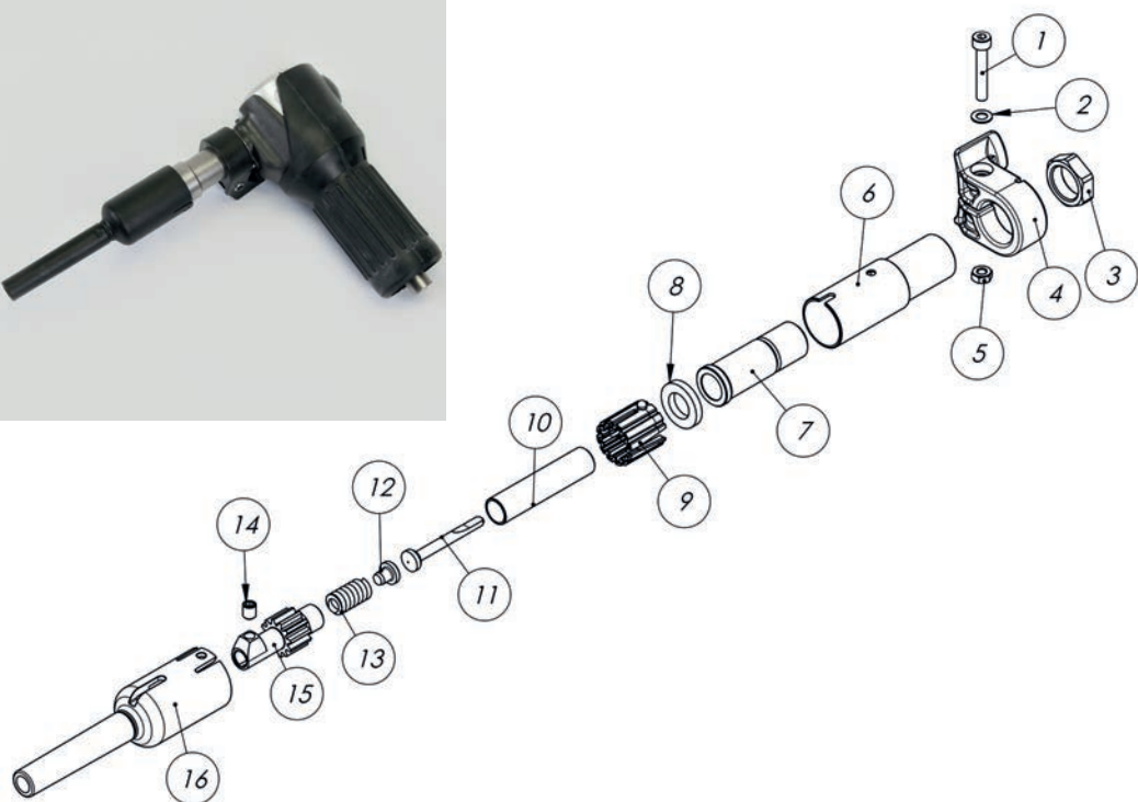
FPM-G brusná hlava
